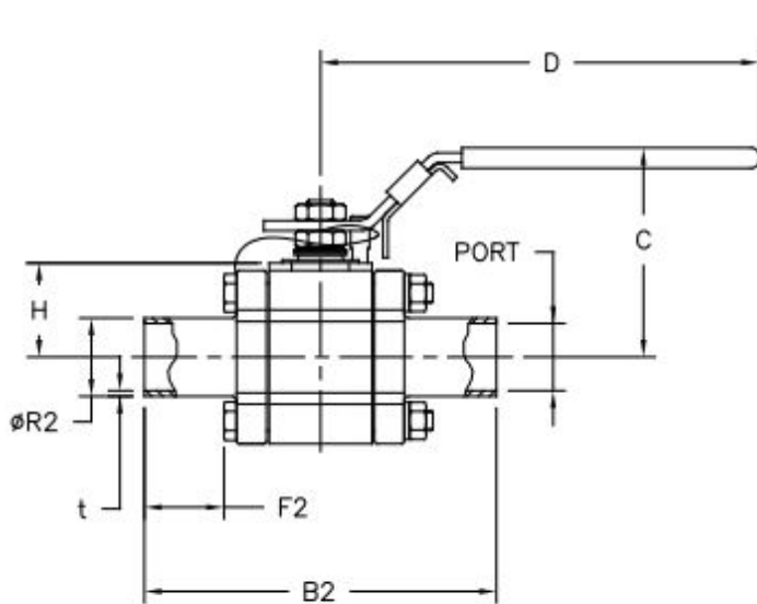
DN15 – DN40
